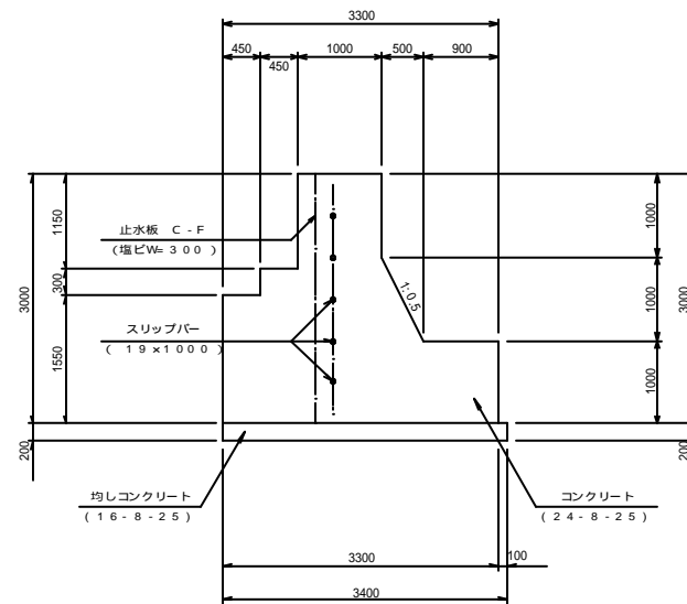
B - B 標準断面図
