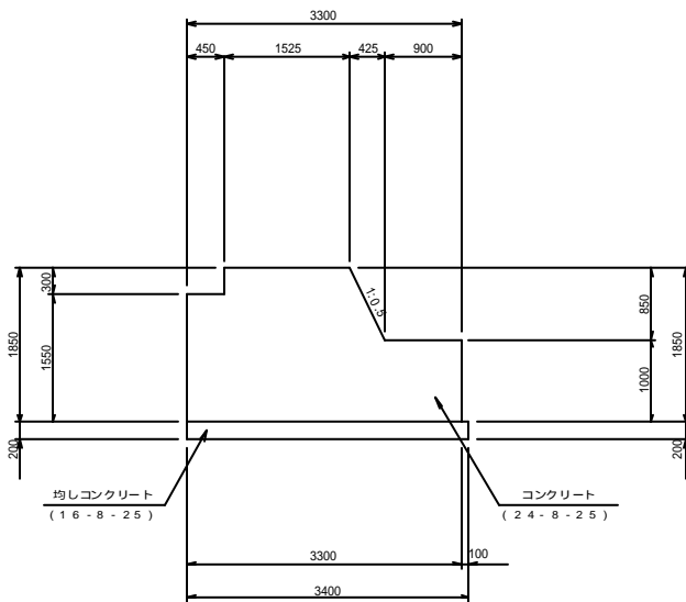
A - A 標準断面図
