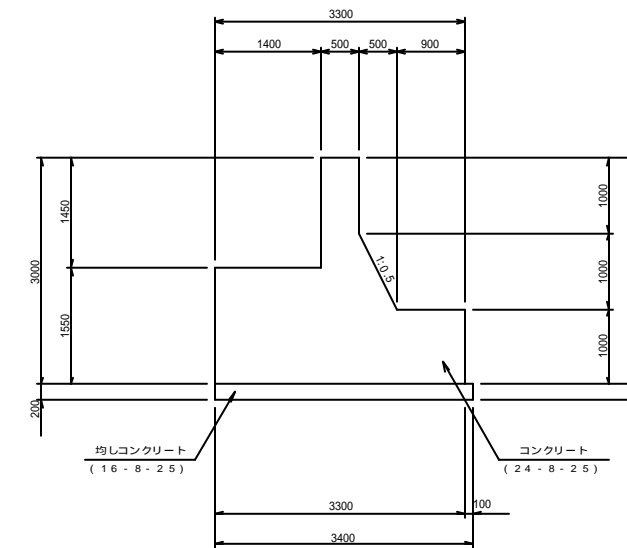
C - C 標準断面図
