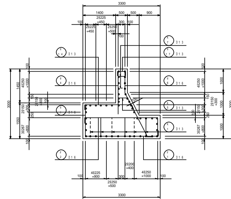
C - C 標準断面図
